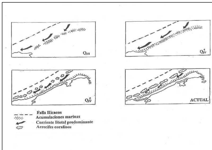
Figura 2. Evolución cuaternaria de la Península de Hicacos.
